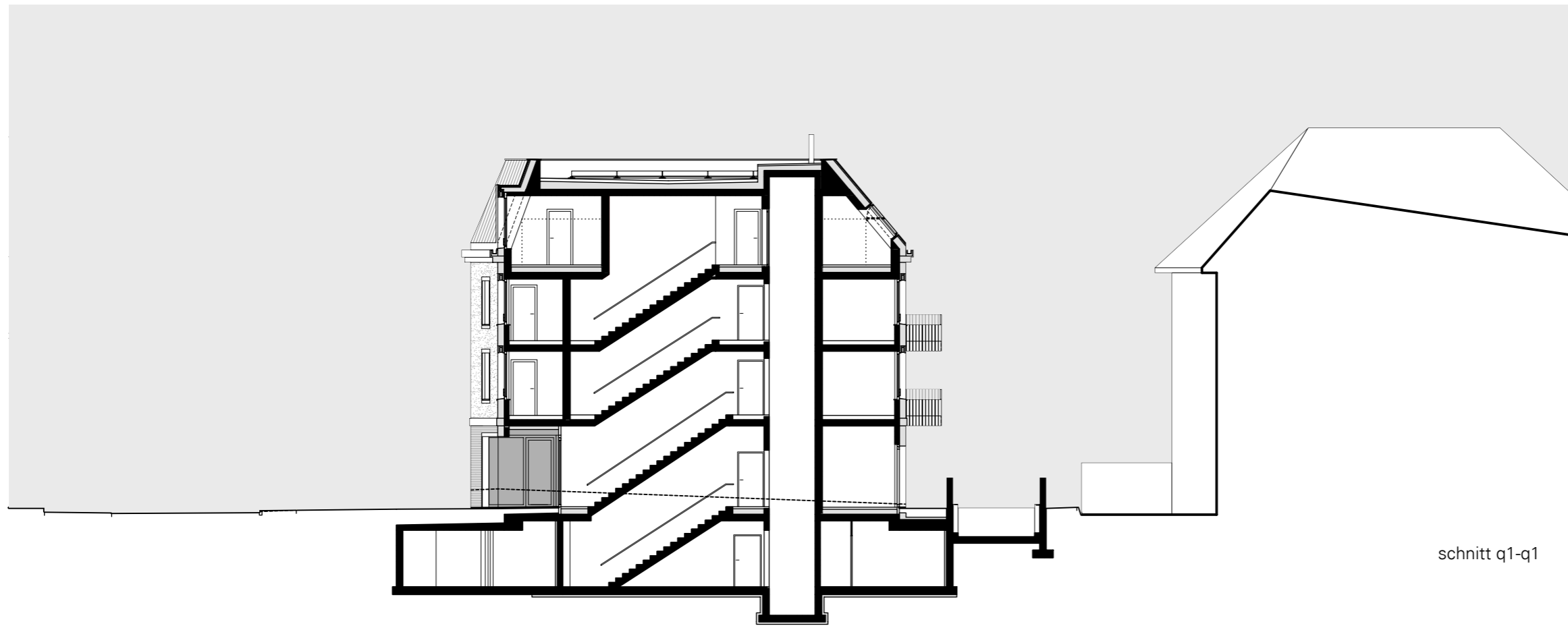
wohnanlage jahnstraße 6, lustenau schnitt q1-q1 schnitt q2-q2
